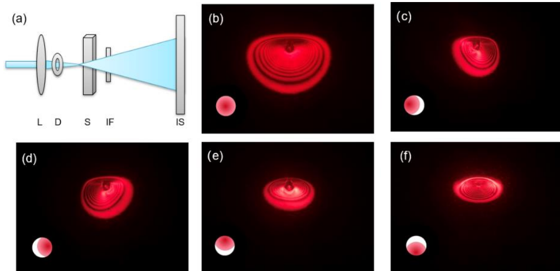
图 S1 光强非高斯分布的激光加热样品时相干环的形状各不相同 (a) 实验装置示意图。白光脉冲光纤激光器经透镜聚焦(L)后通过可变光阑(D)照射在液体样品(S)上, 在成像屏(IS)上形成单色干涉环。样品后方放置了干涉滤光片(IF), 中心波长分别为 632.8 nm (红色)。(b) 激光光轴和可变光阑中心重合时相干环的形状。改变光阑的位置, 分别遮住高斯光束的左半侧(c)、右半侧(d)、上半侧(e)和下半侧(f), 可以让照射到液体里到激光光强变为非高斯分布。(b)-(f)左下角为样品与可变光阑的相对位置示意图
