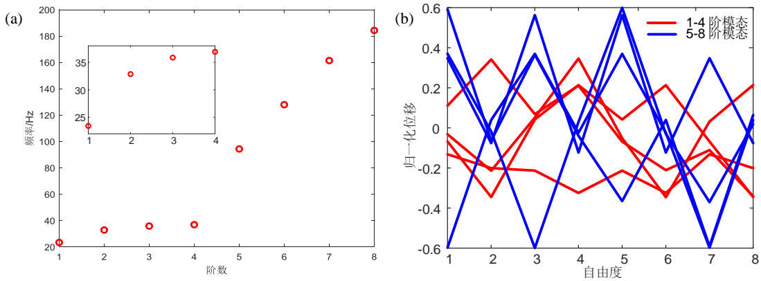
图 S1 波阻隔振器离散模型的 8 阶特征频率和模态向量
