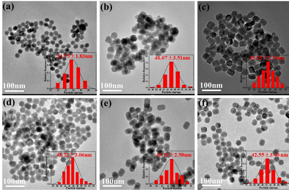
图 S2 (a) \text{NaYF}_4:20\% \text{Yb}^{3+}/12\% \text{Ce}^{3+}/2\% \text{Ho}^{3+} 纳米晶体, (b)–(e) \text{NaYF}_4:20\% \text{Yb}^{3+}/12\% \text{Ce}^{3+}/2\% \text{Ho}^{3+} @ \text{NaYF}_4:x\% \text{Yb}^{3+} ( x=0, 5, 10, 15 )核壳纳米晶体和(f) \text{NaYF}_4:20\% \text{Yb}^{3+}/12\% \text{Ce}^{3+}/2\% \text{Ho}^{3+} @ \text{NaYF}_4:15\% \text{Yb}^{3+}/10\% \text{Nd}^{3+} 核壳纳米晶体的 TEM 图, 插图分别为相应的粒径尺寸分布图
