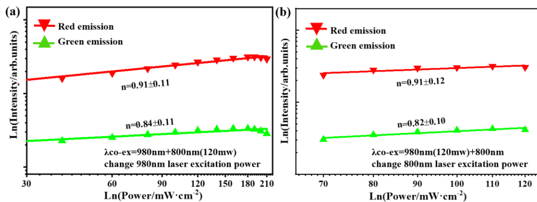
图 S4 在 980 nm 和 800 nm 共同激发下， \text{NaYF}_4:20\% \text{Yb}^{3+}/12\% \text{Ce}^{3+}/2\% \text{Ho}^{3+} @ \text{NaYF}_4:15\% \text{Yb}^{3+}/20\% \text{Nd}^{3+} 核壳纳米晶体红色和绿色荧光强度分别与(a) 980 nm 激光功率的依赖关系和(b)800 nm 激光功率的依赖关系
