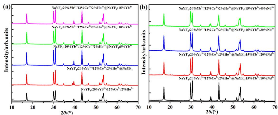
图 S1 (a) \text{NaYF}_4:20\% \text{Yb}^{3+}/12\% \text{Ce}^{3+}/2\% \text{Ho}^{3+} 纳米晶体和 \text{NaYF}_4:20\% \text{Yb}^{3+}/12\% \text{Ce}^{3+}/2\% \text{Ho}^{3+}@/\text{NaYF}_4:x\% \text{Yb}^{3+} ( x = 0, 5, 10, 15 ) 核壳纳米晶体, (b) \text{NaYF}_4:20\% \text{Yb}^{3+}/12\% \text{Ce}^{3+}/2\% \text{Ho}^{3+}@/\text{NaYF}_4:15\% \text{Yb}^{3+}/x\% \text{Nd}^{3+} ( x = 10, 20, 30, 40 ) 核壳纳米晶体的 XRD 图
